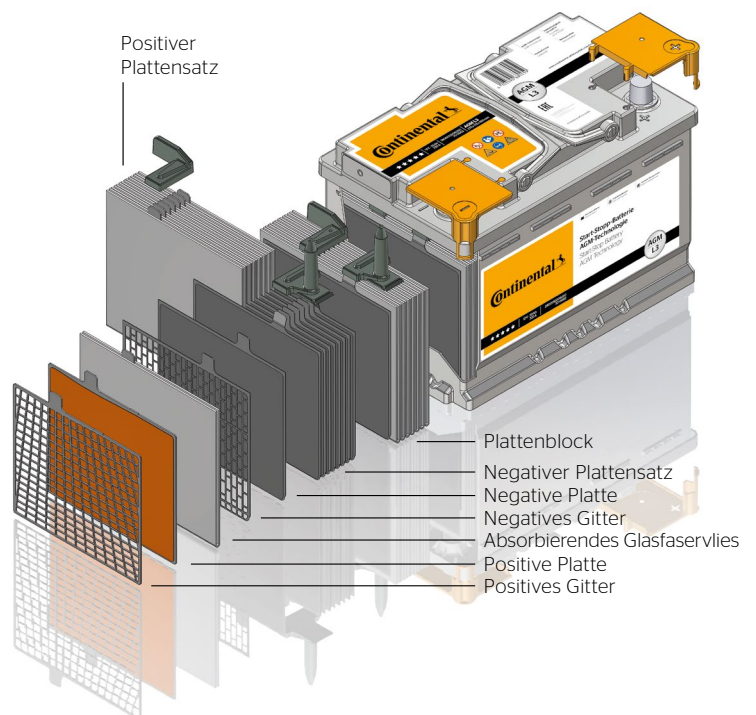
AGM-Technologie: Batterieaufbau
